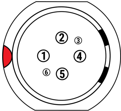
Figure: 雄性6针1B直流电源输入连接器的正面(看着相机的背面)。
