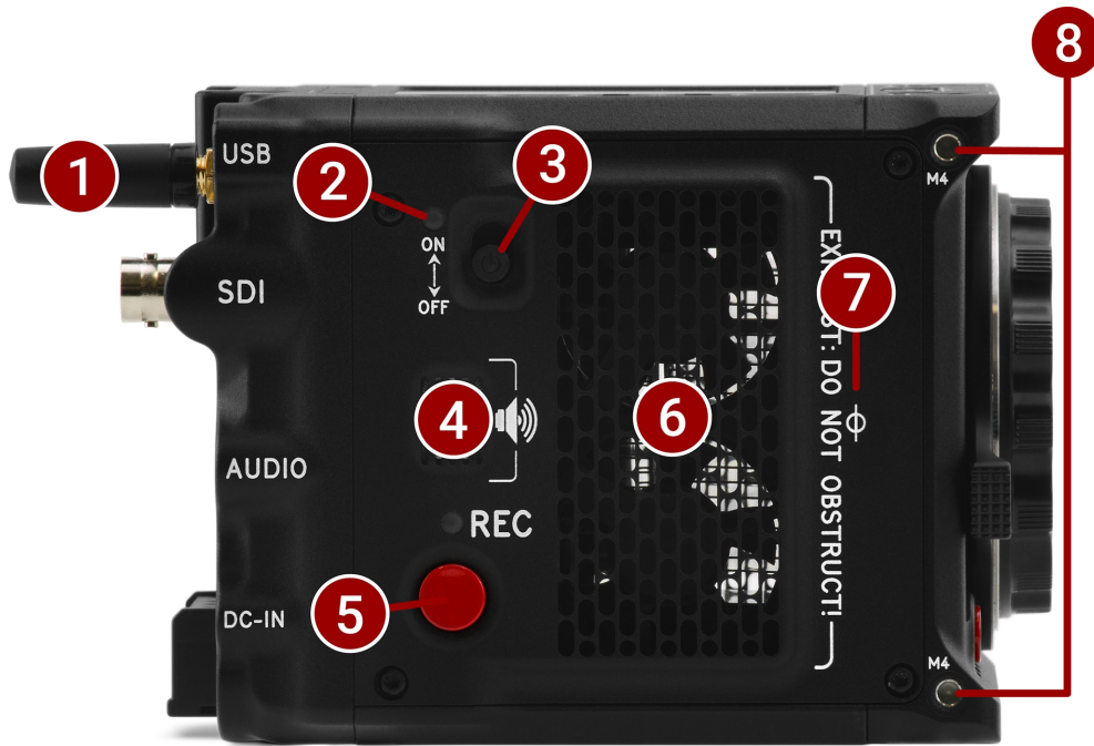
Figure: 相机机身右侧的控制和功能
