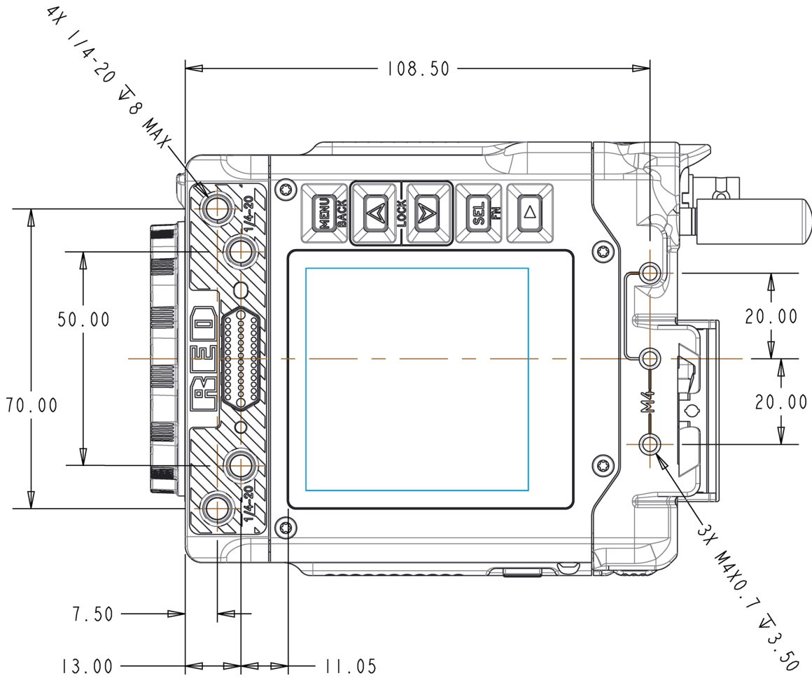
Figure: 摄像机俯视图
