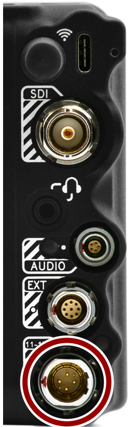
Figure: 雄性6针1B直流电源输入连接器的正面(看着相机的背面)。
