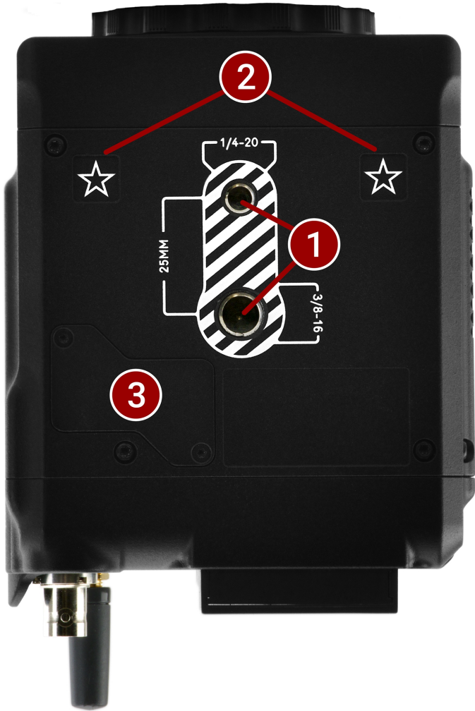
Figure: 相机机身底部控制和功能
