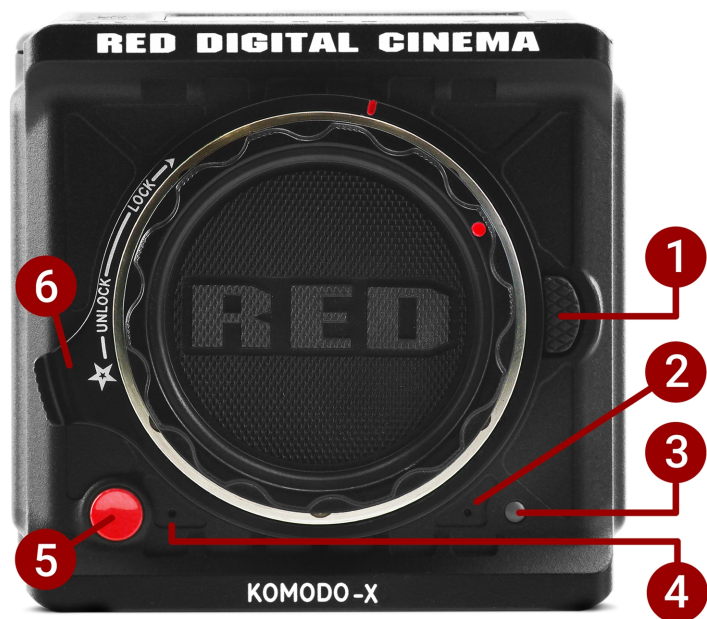
Figure: 相机机身前部控制和功能
