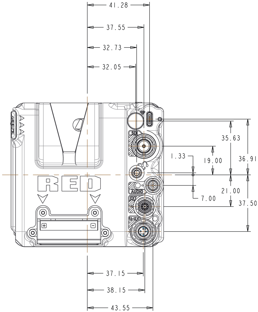
Figure: 摄像机后视图
