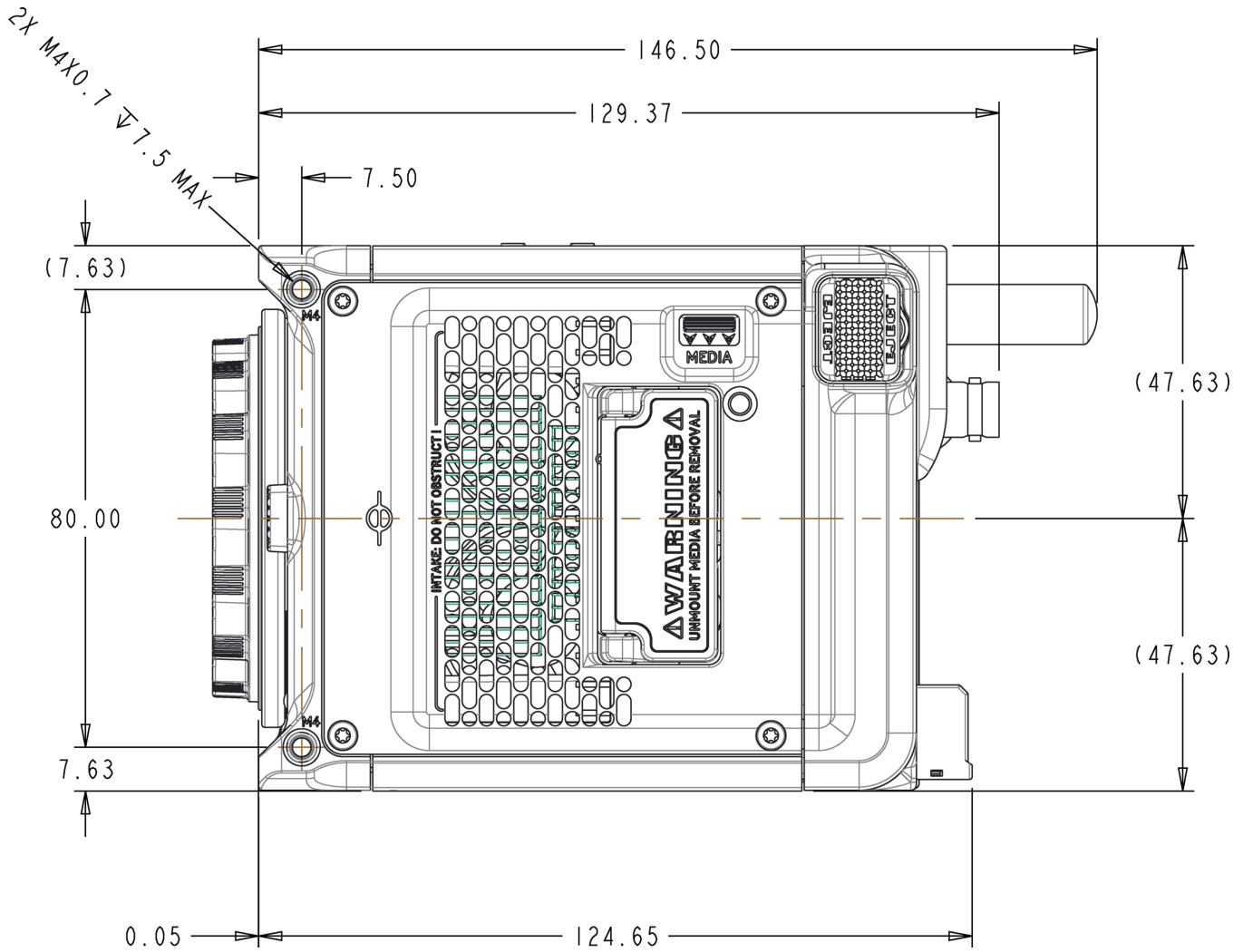
Figure: 相机侧视图(左)
