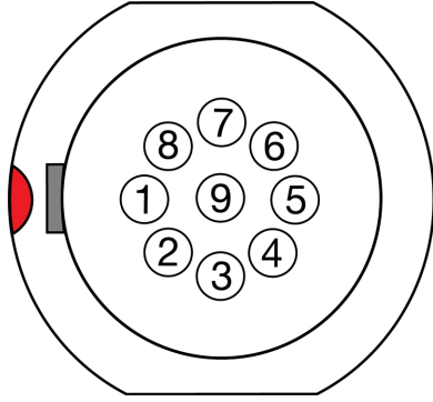
Figure: 雌性9触点扩展端口的正面 (看着相机的背面)。
