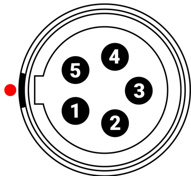
Figure: 雌性5针00B音频连接器的正面(看着相机的背面)。
