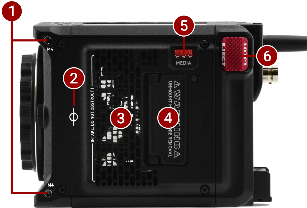
Figure: 相机机身左侧控制和功能
