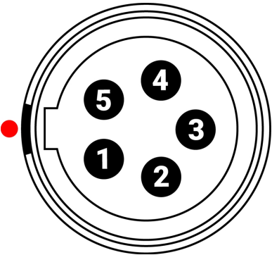
CF: 图: 雌性5针00B音频连接器的正面( 看着相机的背面) 。
