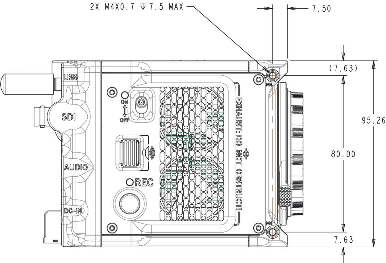
CF:图:相机右侧视图, 射频
