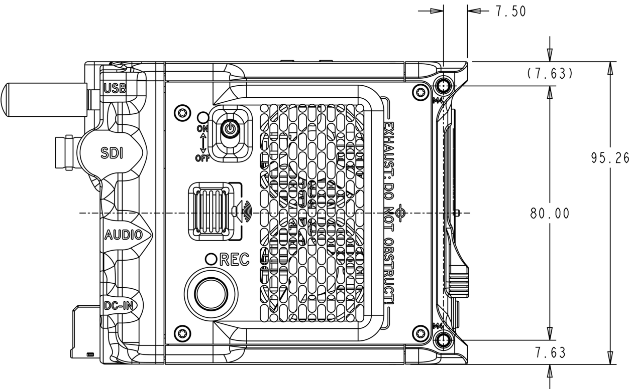
CF:图:相机右侧视图, Z卡口
