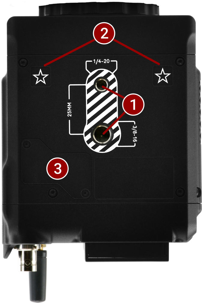
CF:图:相机机身底部控制和功能
