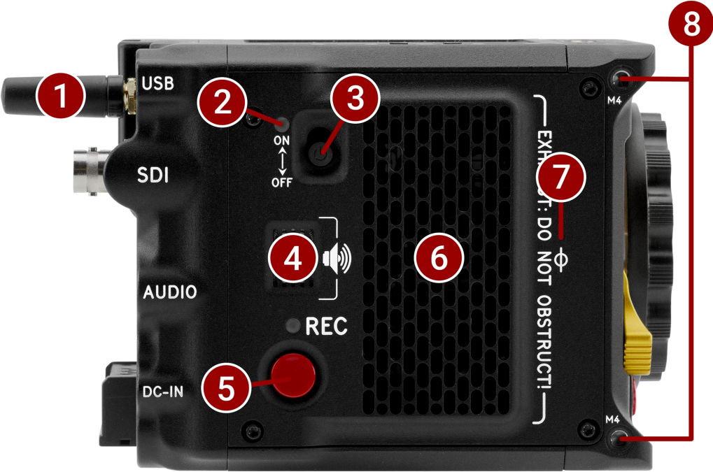
CF:图:相机机身右侧的控制和功能
