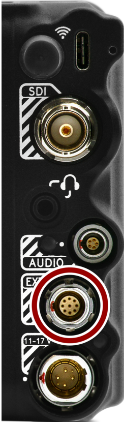
CF:图:雌性9触点扩展端口的正面( 看着相机的背面) 。
