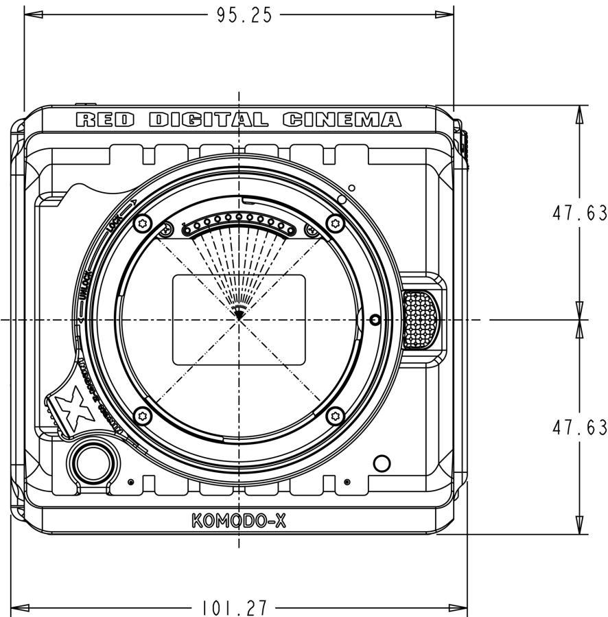
CF:图:相机正面视图,Z卡口
