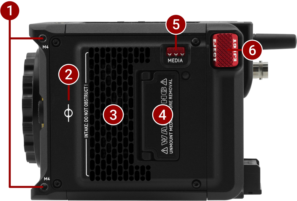
CF:图:相机机身左侧控制和功能
