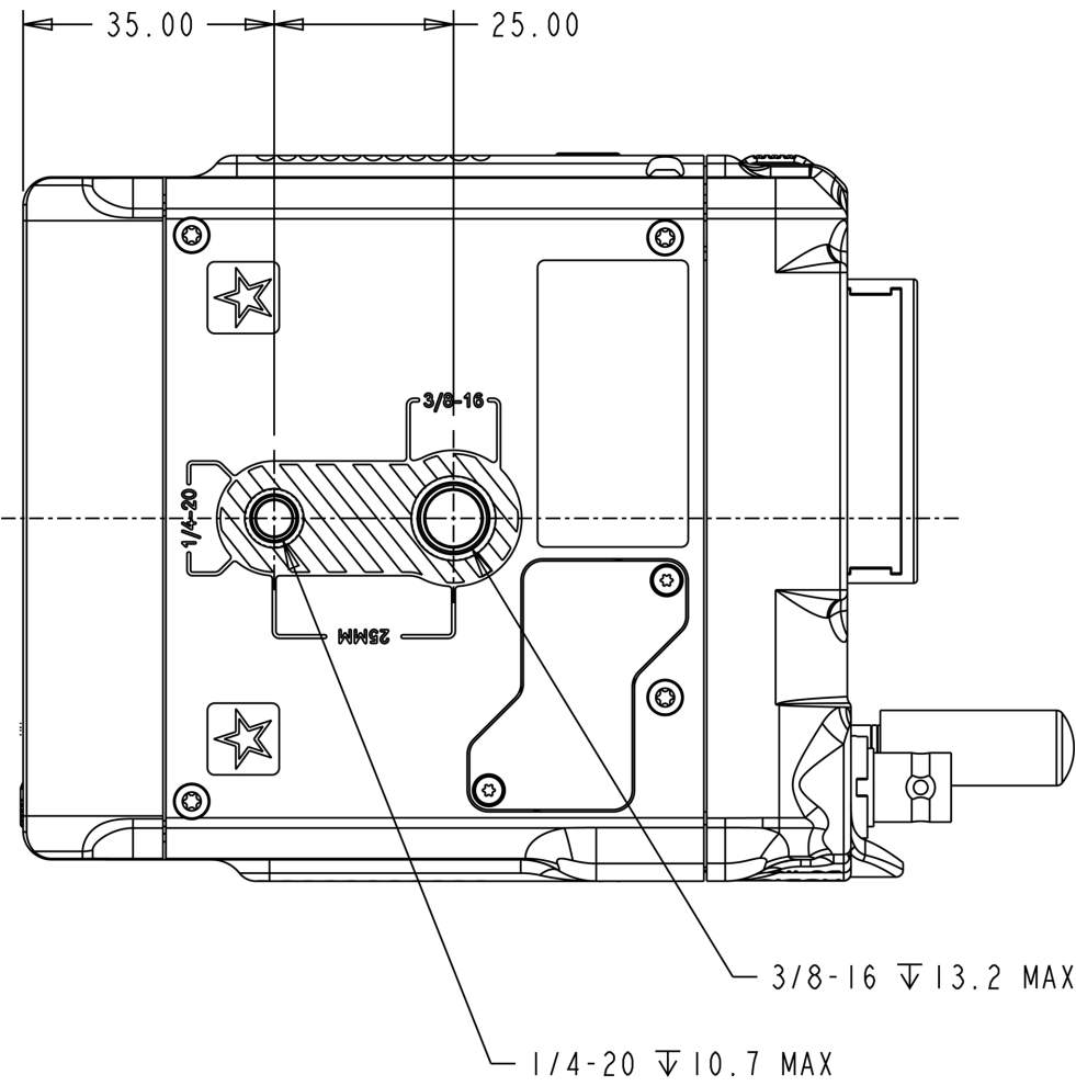
CF:图:相机底部视图,Z轴卡口
