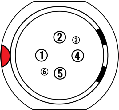
CF:图:雄性6针1B直流电源输入连接器的正面(看着相机的背面)。
