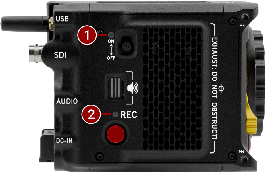
CF:图:摄像头LED, 右侧
