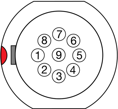
CF:图:雌性9触点扩展端口的正面( 看着相机的背面) 。
