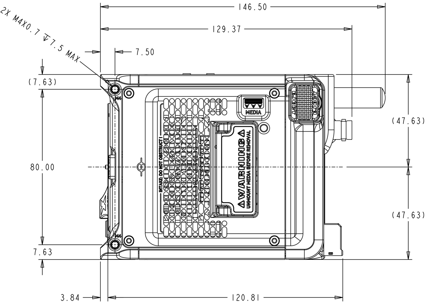
CF:图:相机左侧视图,Z卡口
