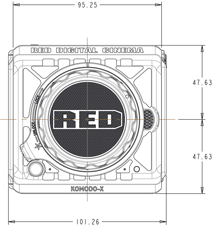
CF:图:摄像头正面视图, 射频
