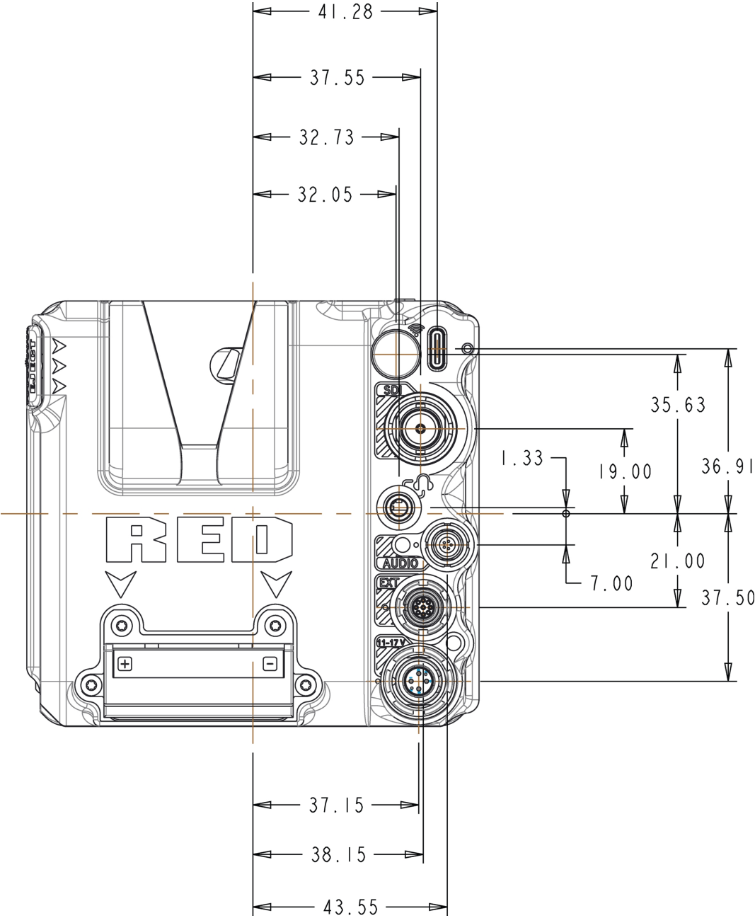
CF:图:摄像头后视图, 射频
