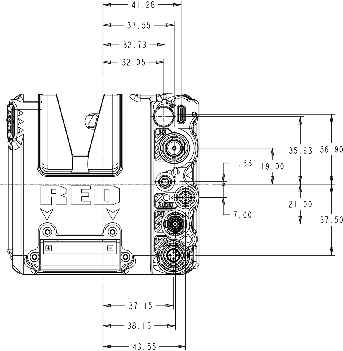
CF:图:相机背面视图,Z卡口
