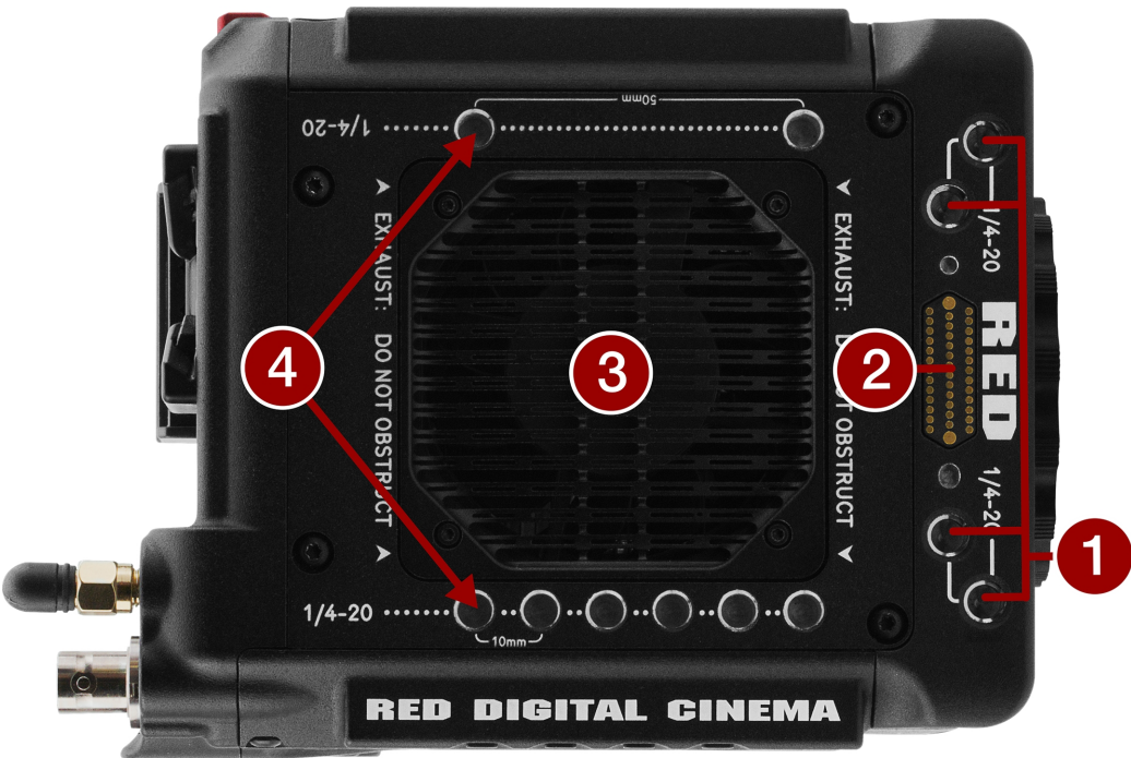
CF:图:相机机身顶部控制和功能
