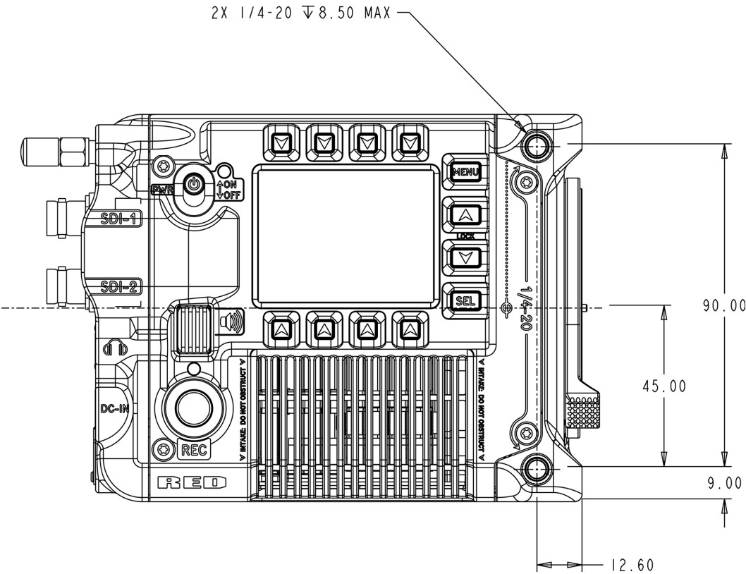
CF:图:相机侧视图(右)。
