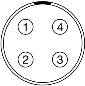
CF:图:4针00B母头CTRL连接器的正面(从连接器正面看)。
