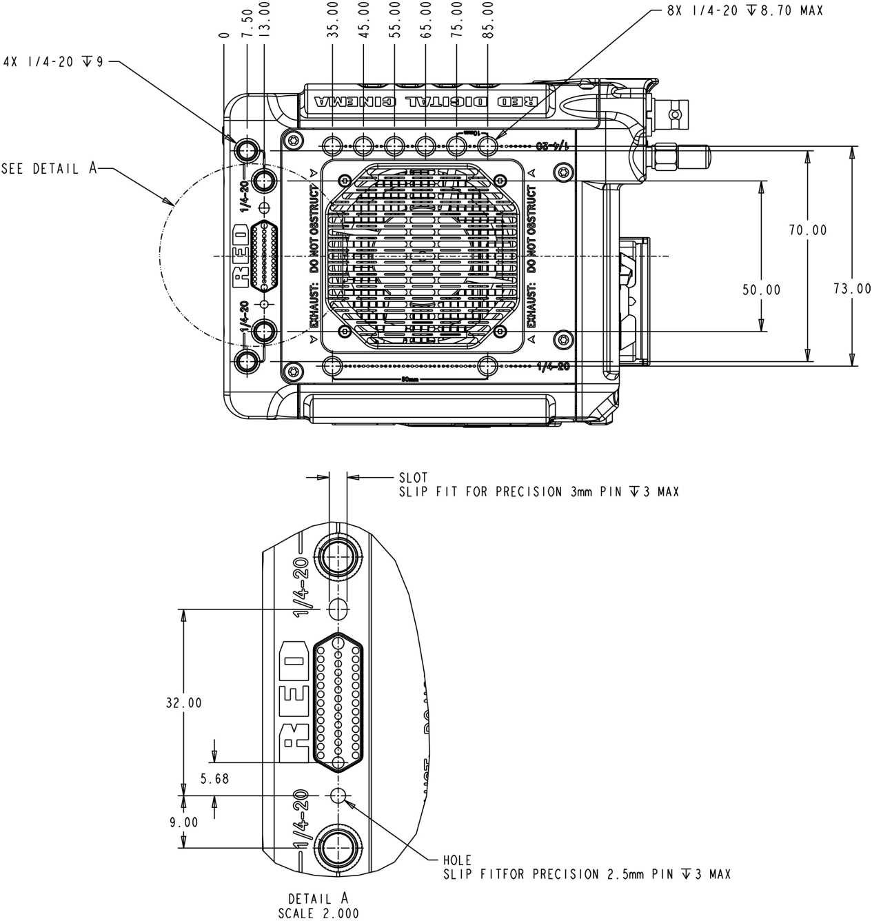
CF:图:摄像机俯视图
