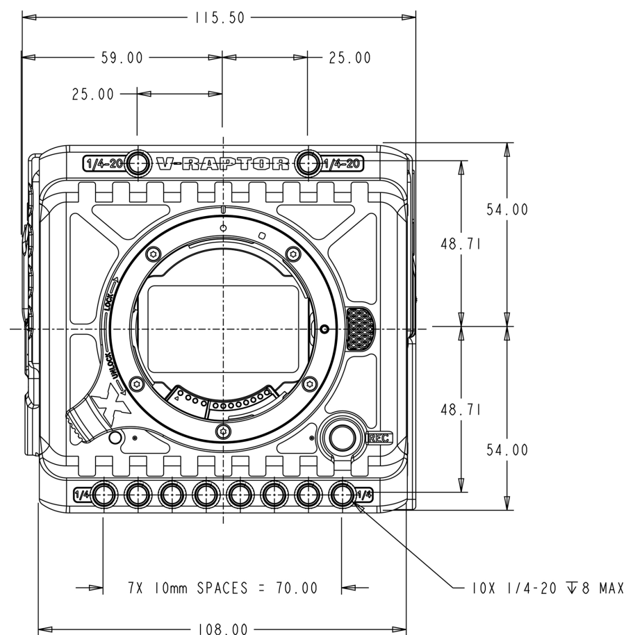
CF:图:摄像机前视图
