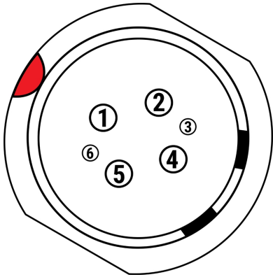
CF: 图: 雄性6针1B直流电源输入连接器的正面( 看着相机的背面) 。
