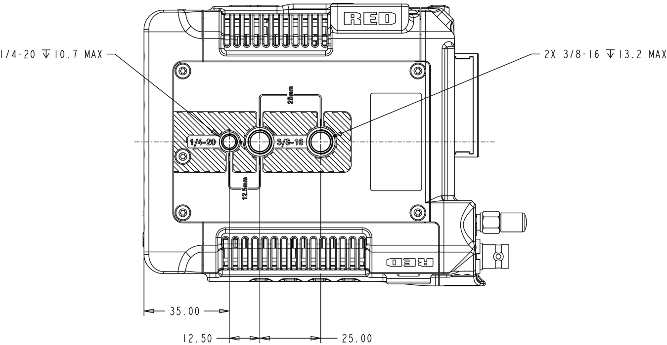
CF:图:摄像机底视图
