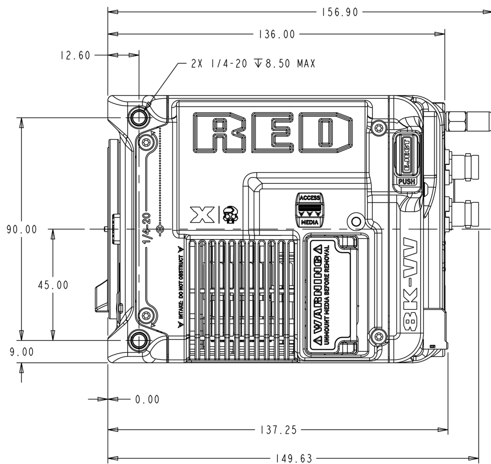
CF:图:相机侧视图(左)
