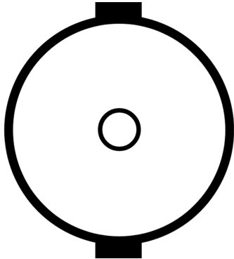
CF:图:12G-SDI公头BNC连接器的正面(看着摄像机的背面)。
