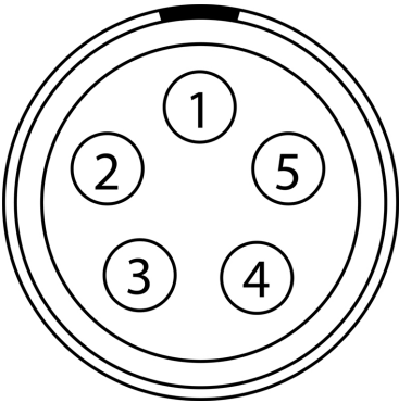
CF:图:时间码 0B 连接器的正面( 从连接器正面看)。
