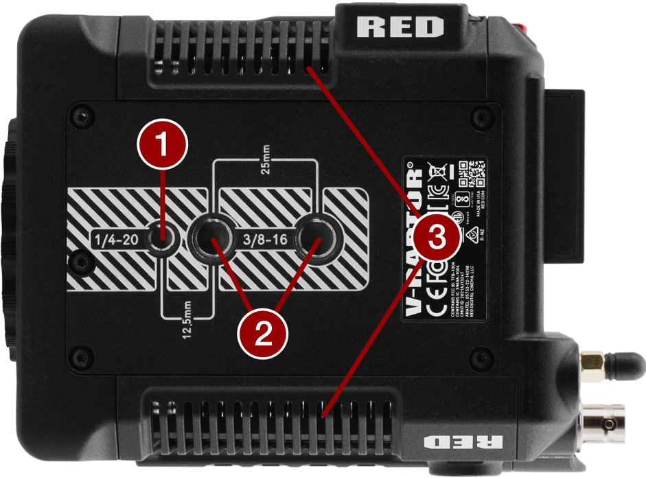
CF:图:相机机身底部特征
