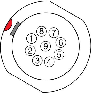
CF: 图: 雌性 9 触点扩展端口的正面 (看着相机的背面)。
