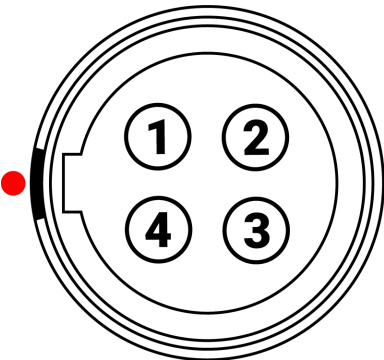
CF: 图: 雄性DC-IN电源输入连接器的正面( 看着相机的背面) 。
