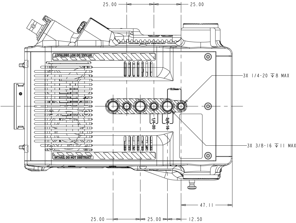
CF:图:摄像机底视图
