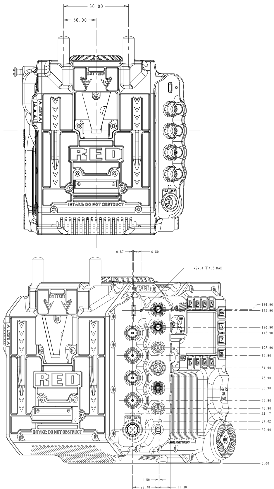
CF:图:摄像机后视图(V型锁)
