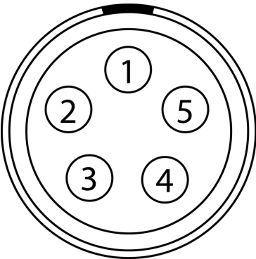
CF: 图:时间码0B连接器的正面( 看着摄像机的背面) 。
