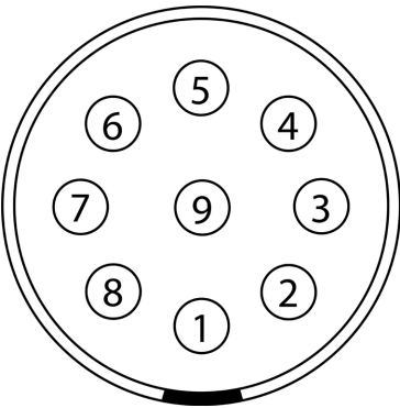
CF: 图:GIG-E连接器的正面( 看着相机的背面) 。
