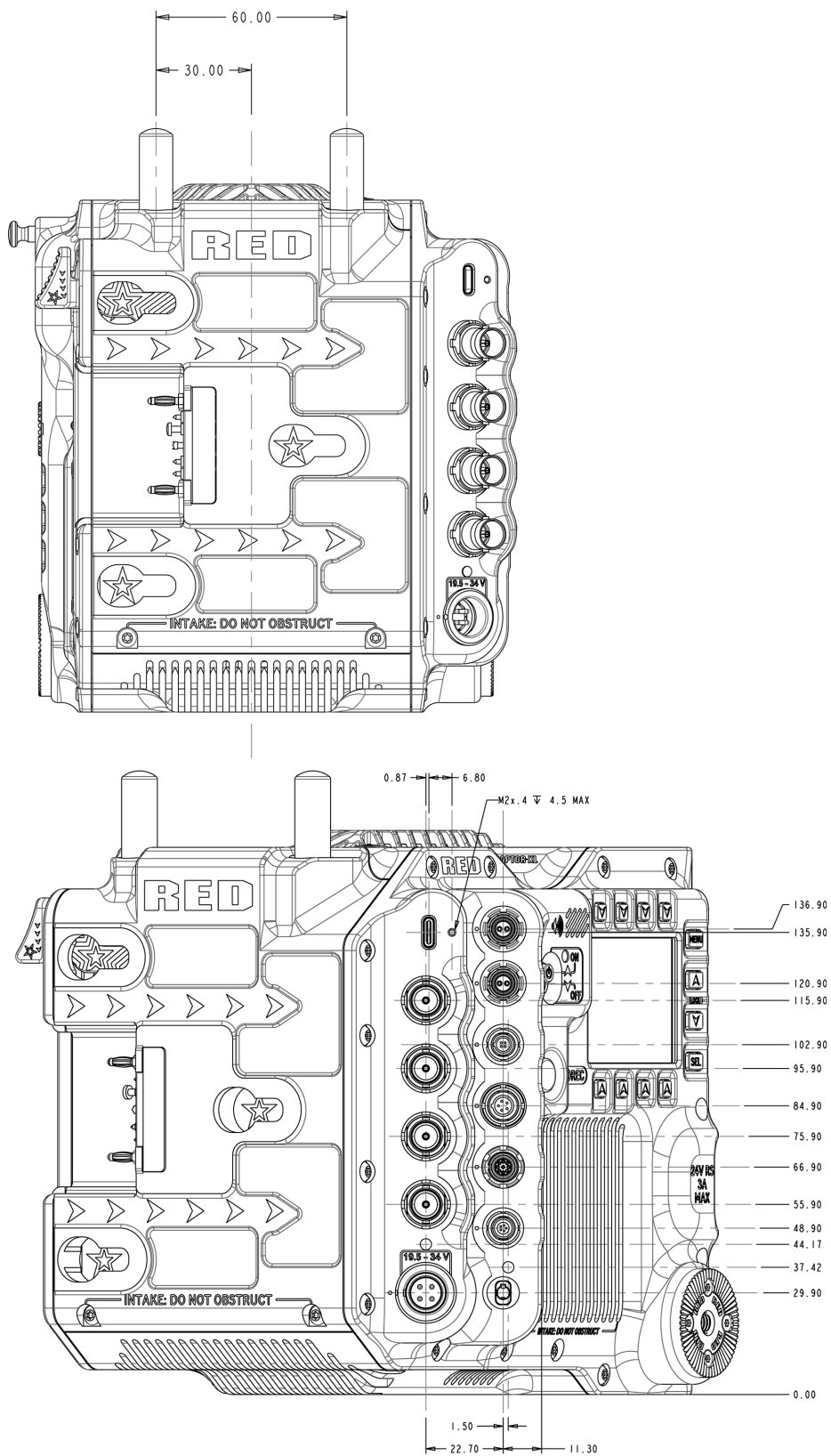
CF:图:摄像机背面图(金装)
