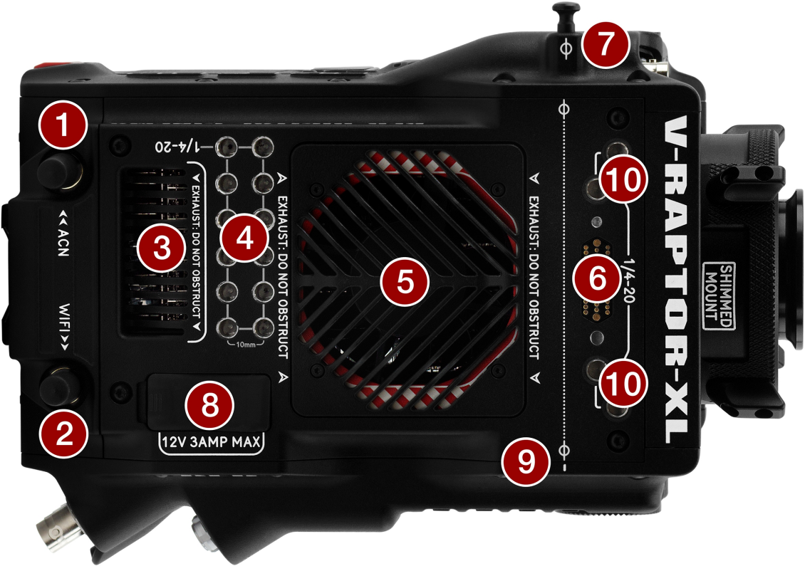
CF: 图: 相机机身顶部、控制和功能
