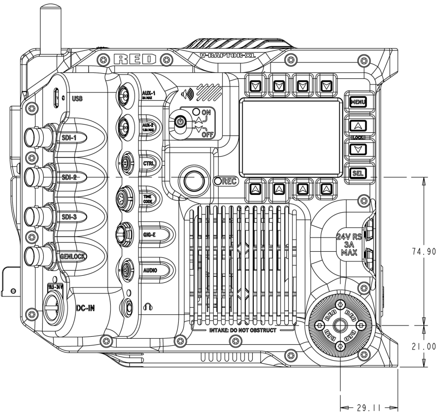
CF:图:相机侧视图( 右) 。
