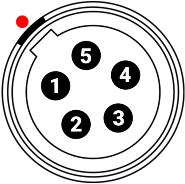
CF: 图: 雌性 5 针 00B 音频连接器的正面( 看着相机的背面) 。
