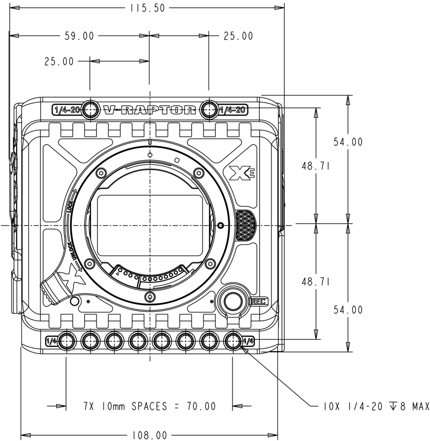
CF:图:摄像机前视图
